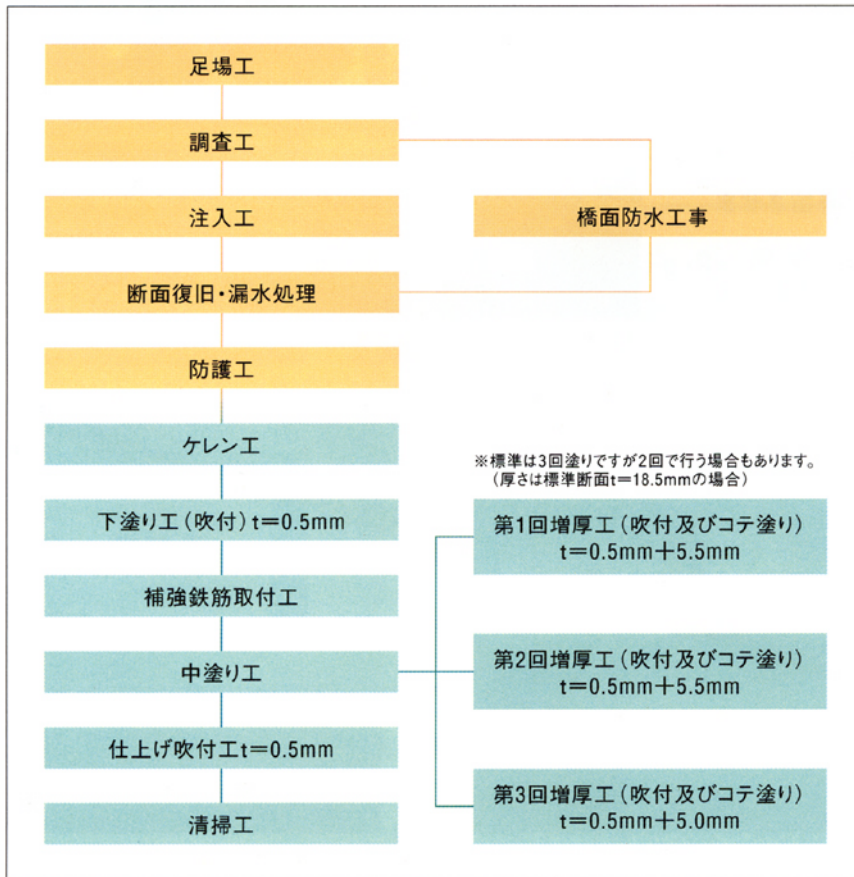
PSR工法の施工フロー図
