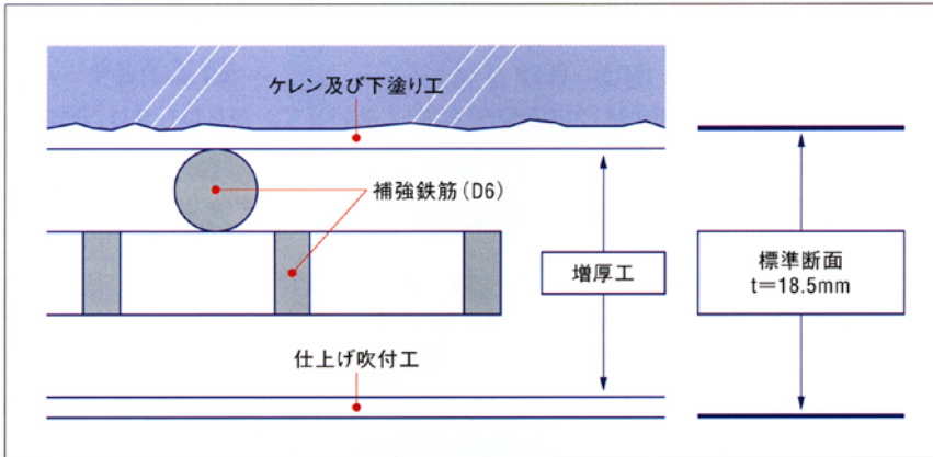
PSR工法 標準施工断面図
